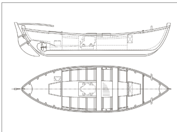
Plano de disposición general de un barquillo de dos proas de Fuerteventura con propulsión intraborda.
